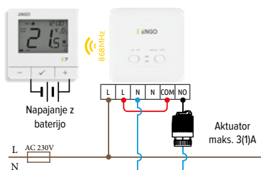
c) Sheme ožičenja za aktuator
