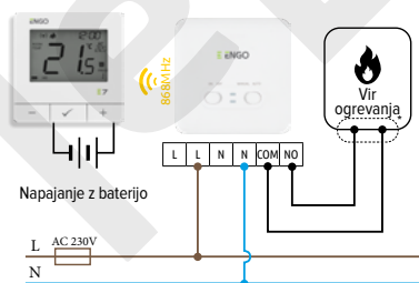
a) Sheme povezave na vir toplote
