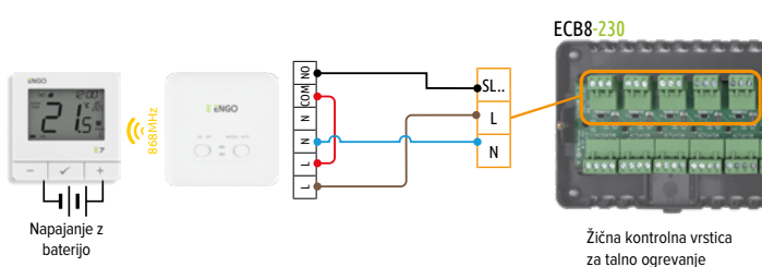
d) Shema povezave za kontrolni trak
