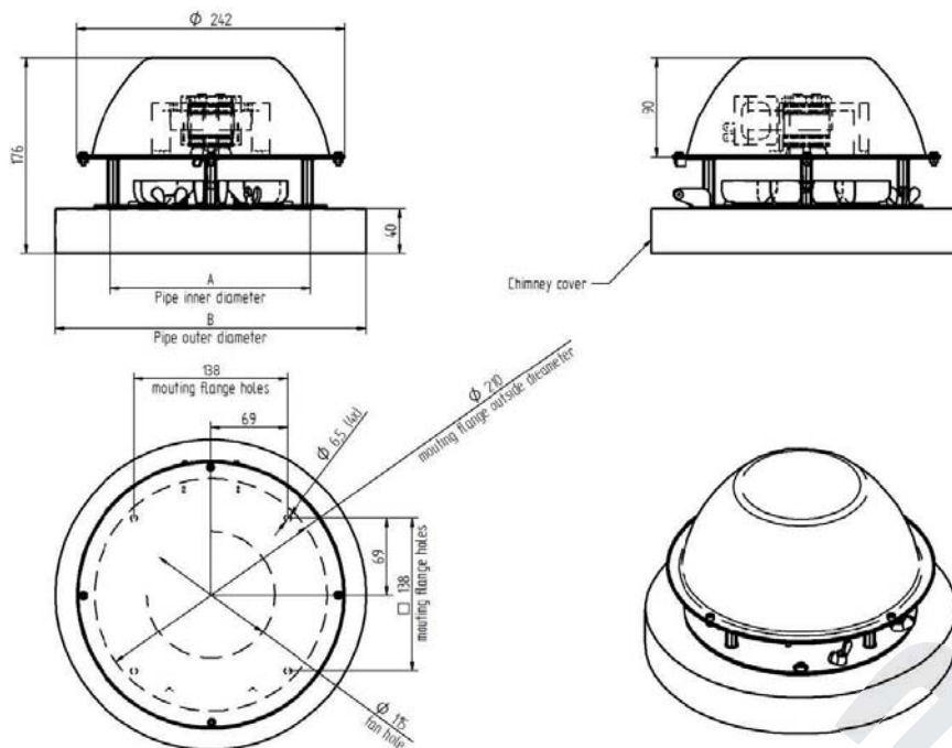
Slika 1 – dimenzije MF0053
