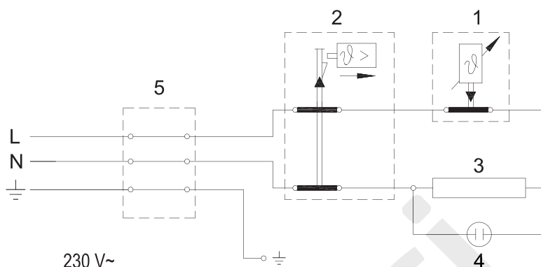
Šema povezivanja električnih provodnika
