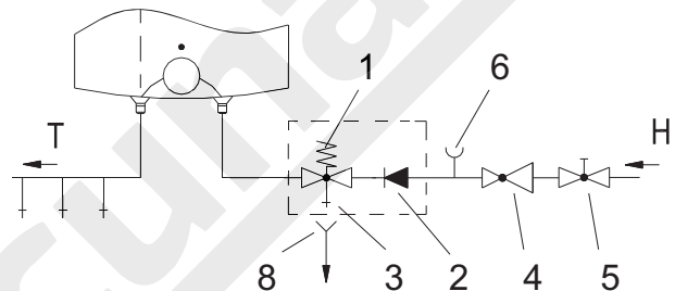
Montage oberhalb des Waschbeckens
