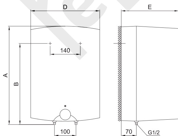
Nadumivalniška izvedba
