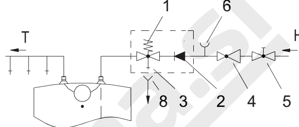
Varijanta ispod umivaonika
