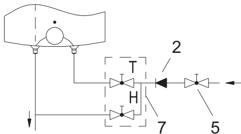
Montage oberhalb des Waschbeckens
