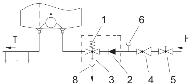
Inačica iznad umivaonika
