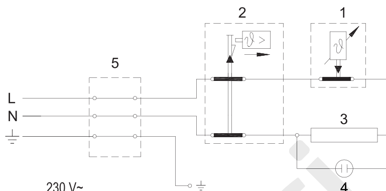
Električna spojna shema
