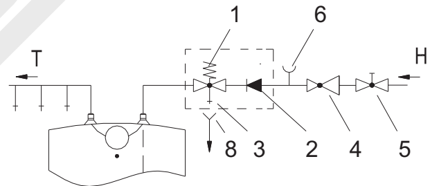
Montage unterhalb des Waschbeckens
