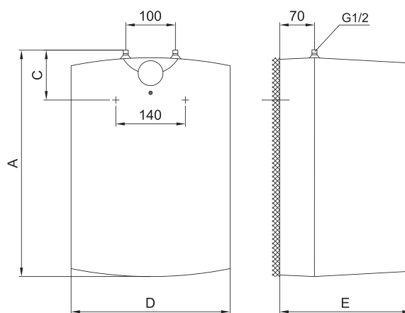
Podumivalniška izvedba
