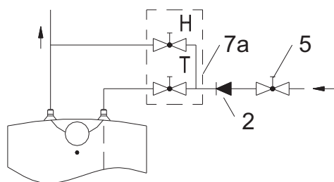
Varijanta ispod umivaonika
