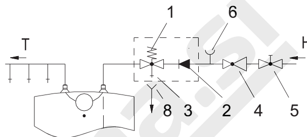
Inačica ispod umivaonika
