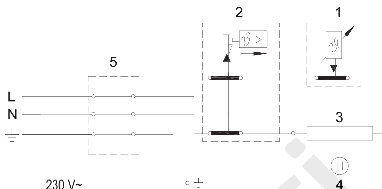
Shema električne vezave
