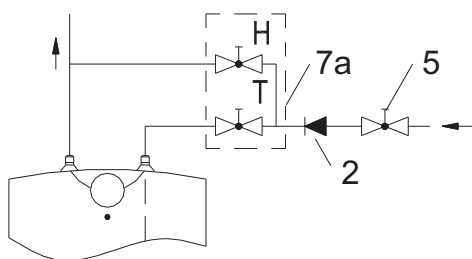
Inačica ispod umivaonika
