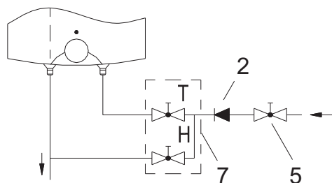
Varijanta iznad umivaonika
