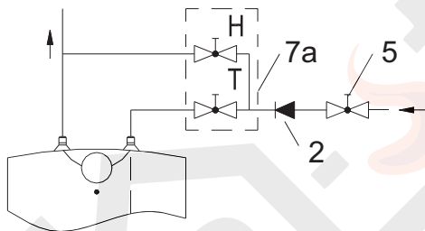
Montage unterhalb des Waschbeckens
