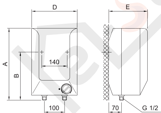
Nadumivalniška izvedba
