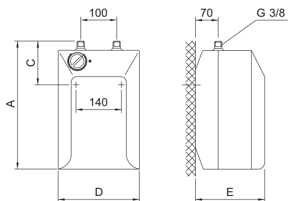
Podumivalniška izvedba
