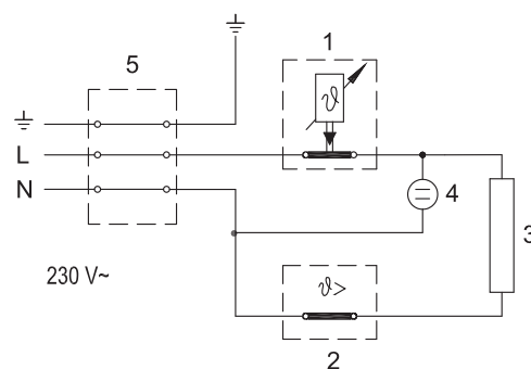
Schema für den Anschluss an die Elektroleitung
