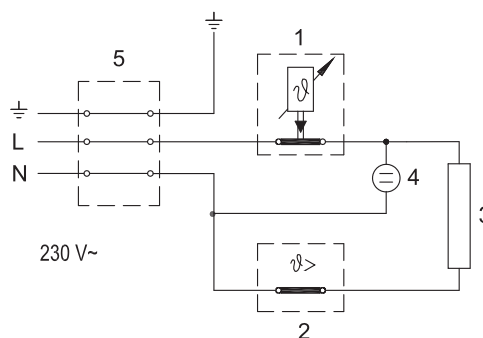
Električna spojna shema
