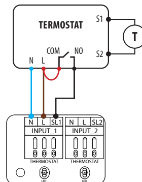
c) Primer diagrama za priklop na razširitveni modul
